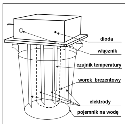
Elektroniczne urządzenie do wody żywej i martwej poj. 4.5l
