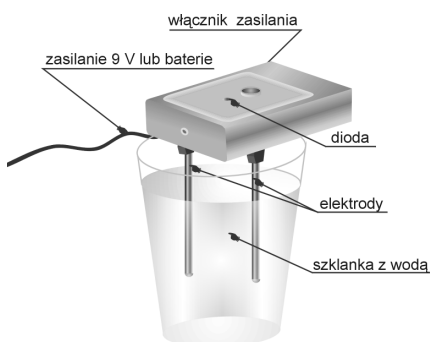
Elektroniczne urządzenie do produkcji srebra, złota, krzemu, cynku koloidalnego, dla pojemności 1/2 litra
